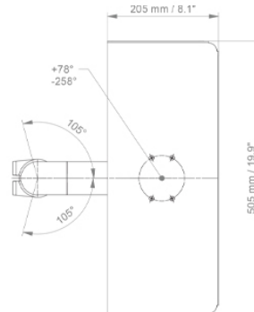
TOP VIEW VUE DE DESSUS - BOVEN BEKIJKEN
