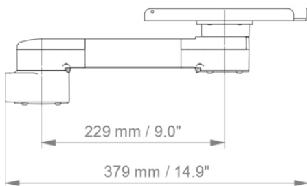
SIDE VIEW - VUE DE CÔTE - ZIJAAZICHT
