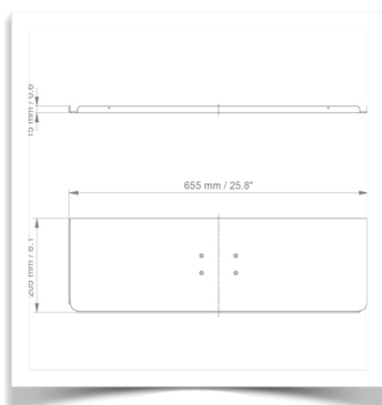
Toetsenbord- en muis houder 655 x 205 mm
