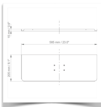
Toetsenbord- en muis houder 585 x 205 mm
