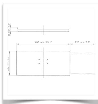
Schuifbare toetsenbord- en muis houder 485 x 220 mm
