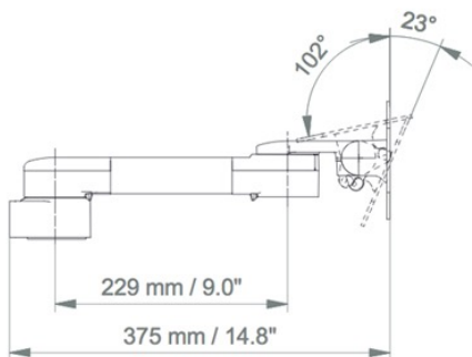
SIDE VIEW - VUE DE CÔTE - ZIJAAZICHT
