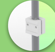
Pince universelle pour tube rond Bride en V pour montage sur tube rond ø 23 - 40 mm
