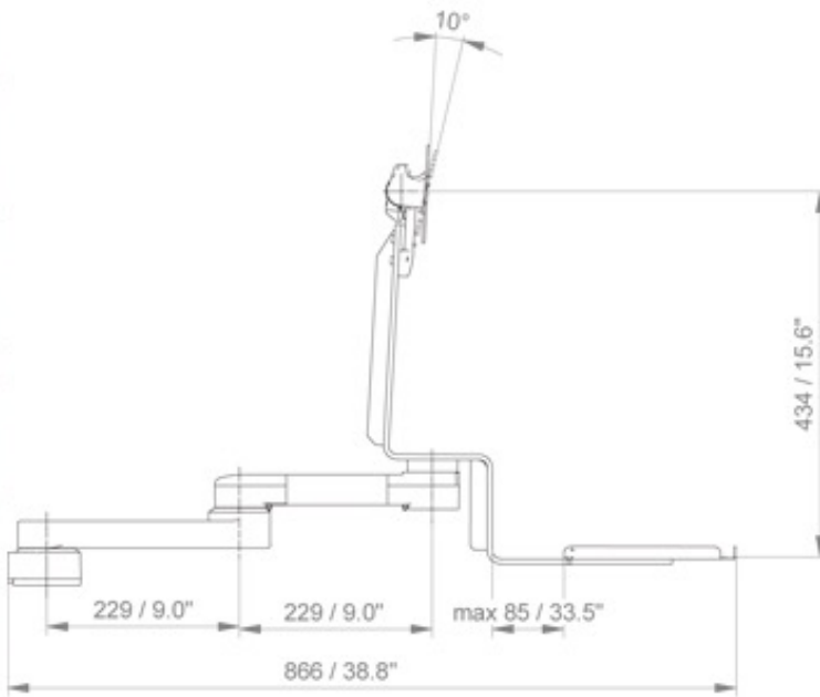
SIDE VIEW - VUE DE CÔTÉ - ZIJAANZICHT
