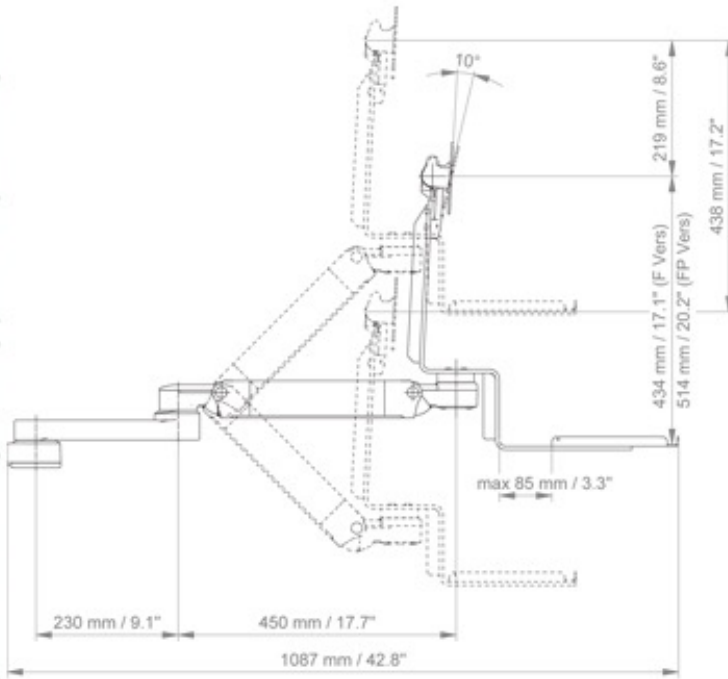
SIDE VIEW - VUE DE CÔTE - ZIJANZICHT
