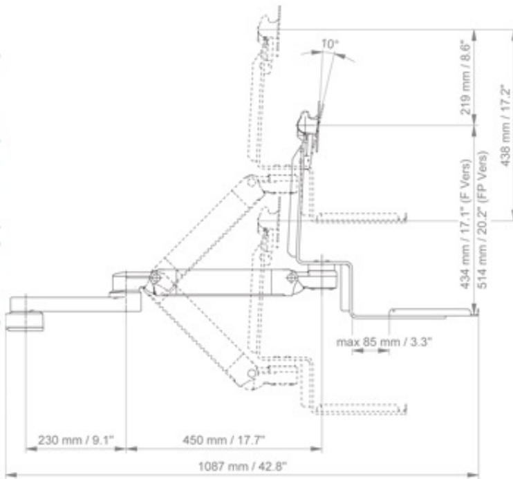
SIDE VIEW - VUE DE CÔTE - ZIJAAANZICHT
