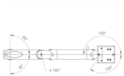
TOP VIEW VUE DE DESSUS - BOVEN BEKIJKEN
