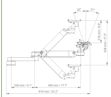
SIDE VIEW - VUE DE CÔTE - ZIJAAANZICHT
