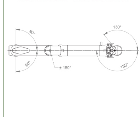
TOP VIEW VUE DE DESSUS - BOVEN BEKIJKEN
