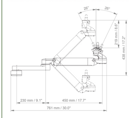
SIDE VIEW - VUE DE CÔTE - ZIJAAZICHT
