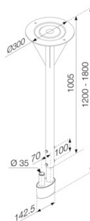
SIDE VIEW - VUE DE CÔTE - ZIJEAANZICHT
